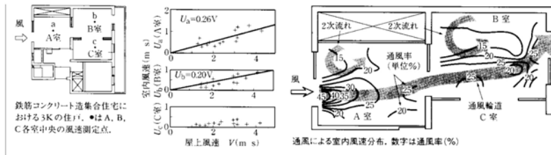
鉄筋コンクリート造集合住宅における3Kの住戸。●はA, B, C各室中央の風速測定点。 屋上風速 V (m/s) と室内風速 U (m/s) の関係 風は風上開口と風下開口を結ぶ線に沿って通風輪道を生じる。そこでの風速は外部の風速に比例し、通風率(=室内風速/外部風速)は一定となる。しかし、間仕切り開口で接する他の通風輪道からはずれる家の風速は、外部の風速に比例せず非常に弱い。通風時の風速分布は複雑であり、通風輪道の風は同じ室内の開放空間に二次気流を生じさせる。
