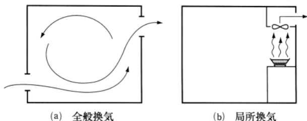
図 全般換気と局所換気（出典：参考文献 [3]，p.17）
