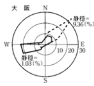
蒸暑季の大阪(5月中旬~10月初旬)と福岡(5月中旬~10月中旬)における時間帯別風配と風速頻度分布 大阪:実線は13:00~18:00、破線は3:00~8:00のデータ。福岡:実線は12:00~18:00、破線は24:00~6:00のデータ
