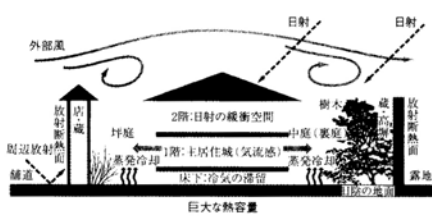
植栽や水面を有して低湿面を形成する二つの中庭の空間ボリュームの違いによって生じる圧力差を利用し、室内に風を発生させ、深い軒庇、葺や高欄によって日射を遮蔽している京都の町家。
