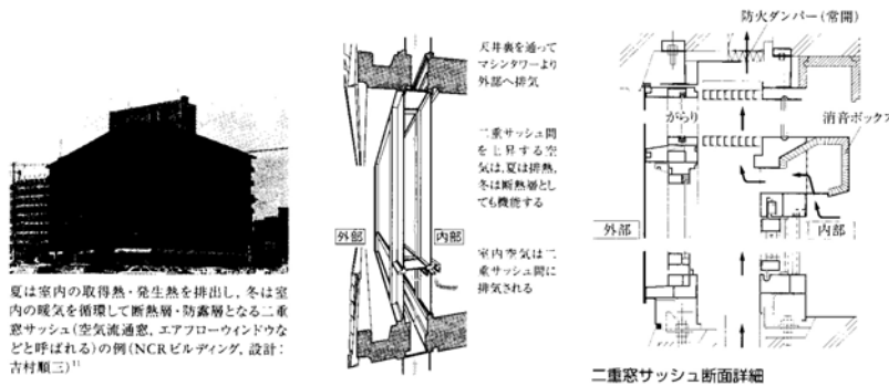
夏は室内の取得熱・発生熱を排出し、冬は室内の暖気を循環して断熱層・防露層となる二重窓サッシ(空気流通窓、エアフローウィンドウなどと呼ばれる)の例(NCRビルディング, 設計: 古村順三) 1) 二重窓サッシ断面詳細
