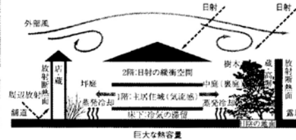
植栽や水面を有して低湿面を形成する二つの中庭の空間ボリュームの違いによって生じる圧力差を利用し、室内に風を発生させ、深い軒庇、蔵や高欄によって日射を遮蔽している京都の町家。
