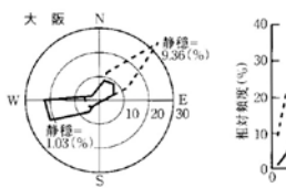
夏季の大阪(5月中旬~10月初旬)と福岡(5月中旬~10月中旬)における時間帯別風配と風速頻度分布 大阪実績は13:00~18:00、破線は3:00~8:00のデータ、福岡実績は12:00~18:00、破線は24:00~6:00のデータ
