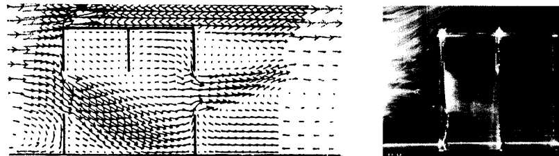
通風の効果は室内の風速分布によってほぼ決定される。間仕切りを有する独立模型内の通風時風速の断面内分布に関し、乱流数値シミュレーションによる風速ベクトル分布と風洞模型実験により可視化したものを比較すると、両者の気流パターンはよく一致している。
