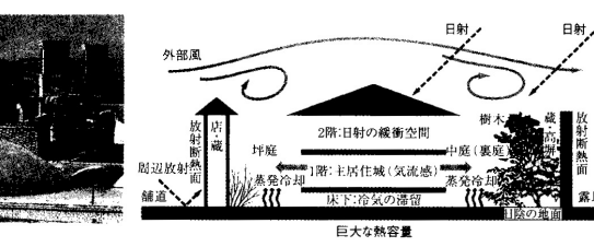
植栽や水面を有して低温面を形成する二つの中庭の空間ボリュームの違いによって生じる圧力差を利用し、室内に風を発生させ、深い軒庇、蔵や高扉によって日射を遮蔽している京都の町家。 19)
