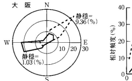
蒸暑季の大阪(5月中旬~10月初旬)と福岡(5月中旬~10月中旬)における時間帯別風配と風速頻度分布 大阪:実線は13:00~18:00、破線は3:00~8:00のデータ、福岡:実線は12:00~18:00、破線は24:00~6:00のデータ
