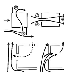
高温多湿地域の開放的な住居。風上と風下で大きな開口を設ける。
