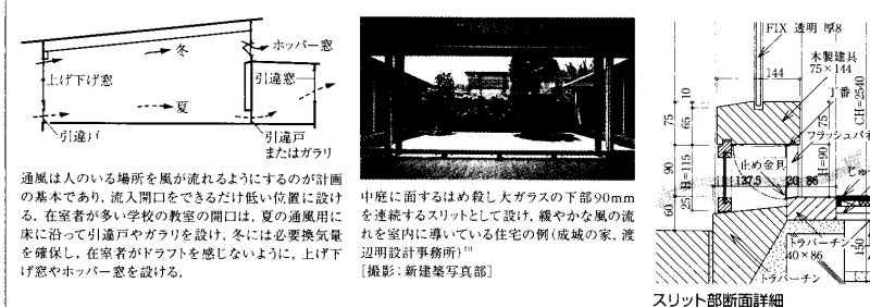
通風率は人のいる場所を風が流れるようにするのが計画の基本であり、流入開口をできるだけ低い位置に設ける。在室者が多い学校の教室の開口は、夏の通風用に床に沿って引違戸やガラリを設け、冬には必要換気量を確保し、在室者がドラフトを感じないように、上げ下げ窓やホッパー窓を設ける。 中庭に面するはめ殺し大ガラスの下部90mmを連続するスリットとして設け、緩やかな風の流れを室内に導いている住宅の例(成城の家、渡辺明設計事務所) [撮影: 新建築写真部]
