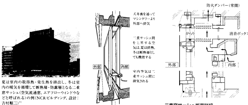
夏は室内の取得熱・発生熱を排出し、冬は室内の暖気を循環して断熱層・防霜層となる二重窓サッシ(空気流通窓、エアフローウィンドウなどと呼ばれる)の例(NCRビルディング, 設計: 吉村順三) 二重窓サッシ断面詳細
