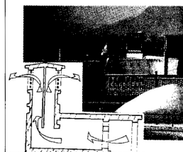
日射で塔が熱せられ、室内の暖かい空気が上昇し、涼しい空気が引き込まれる。高温乾燥地域で換気塔を備え、家の中に風道を作っている例。
