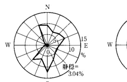
東京における蒸暑季(日平均気温 \geq 20 、5月下旬~10月初旬)は、大洋から大陸に吹き込む季節風と海陸風がよく発達する。風向を時間帯分類すると、早朝風向がより明確になる。季節風と海風の風向が一致する時間帯の風速は、陸寄りの風が吹く時間帯に比較して1.5倍程度大きい。
