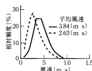
時間帯別の風配と風速頻度分布では、実線が海寄りの風の吹きやすい時間帯(13:00-19:00)、点線が陸寄りの風の吹きやすい時間帯(3:00-9:00)のデータを示す。
