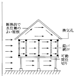
高温多湿地域の開放的な住居。風上と風下で大きな開口を設ける。
