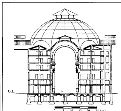
図6 ミラノ内部測定地点断面図
