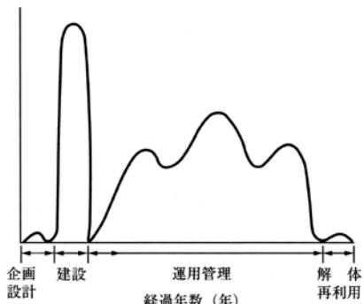
図 LCC 経年支出の概念 (出典：参考文献 [2], p. 148)
