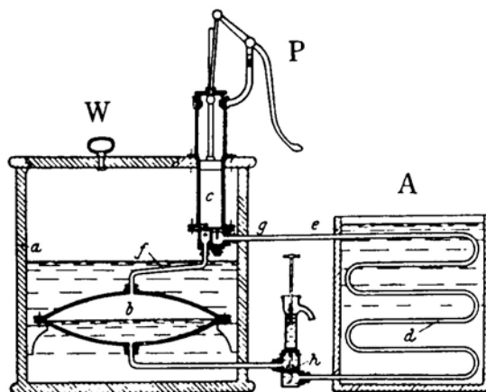
W：コンデンサー，A：エバポレーター（A中の水を氷にすることができる），h：膨張弁
