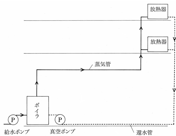
図 ウェブスター式蒸気暖房の模式図
