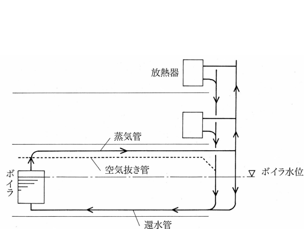
ケルチング式蒸気暖房の模式図
