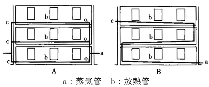
図 同径の铸铁管を連続して用いた一管式蒸気暖房 (参考文献 [9], p. 65)
