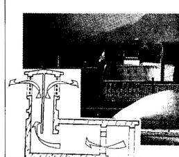
高温多湿地域の開放的な住居。風上と風下で大きな開口を設ける。
