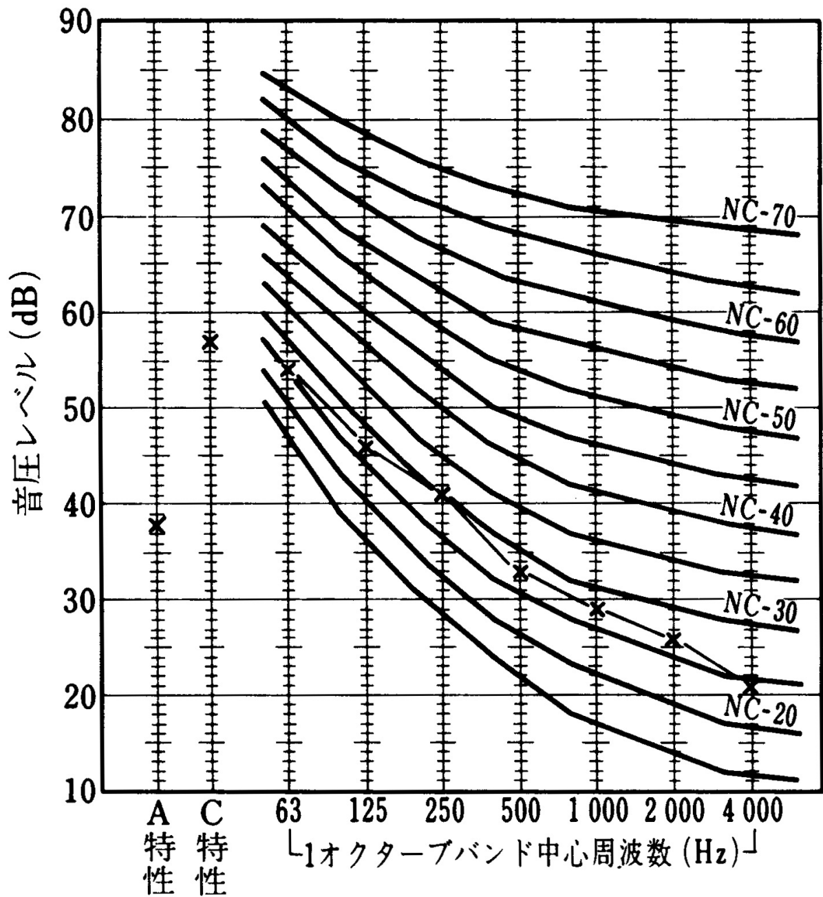
図4.1.4 NC 曲線による室内騒音の評価
