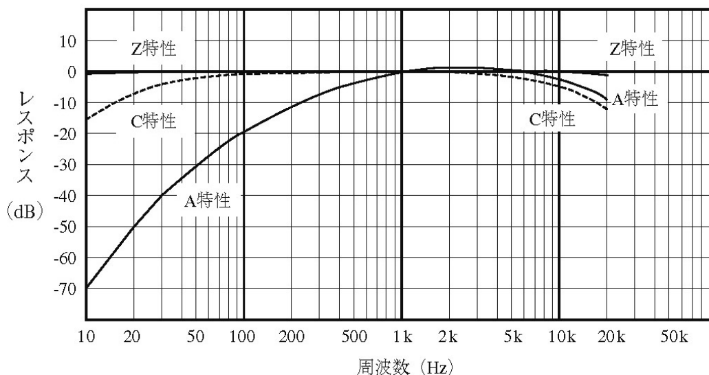
周波数重み付け回路の特性
