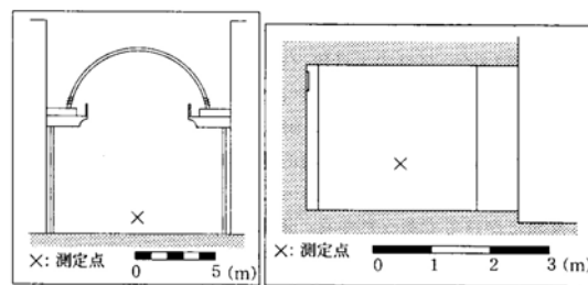
図16 今治の断面図
