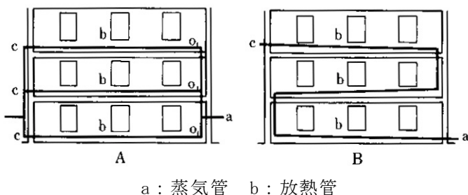
図 同径の鑄鉄管を連続して用いた一管式蒸気暖房 (参考文献 [9], p. 65)
