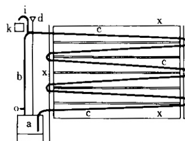
図 ボンネマンの温水暖房 (参考文献 [9], p. 65)
