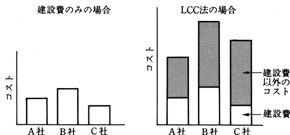
建設費だけ見るとC社が最小であるが、ライフサイクルコストを考えると、実はA社が最小になる。
