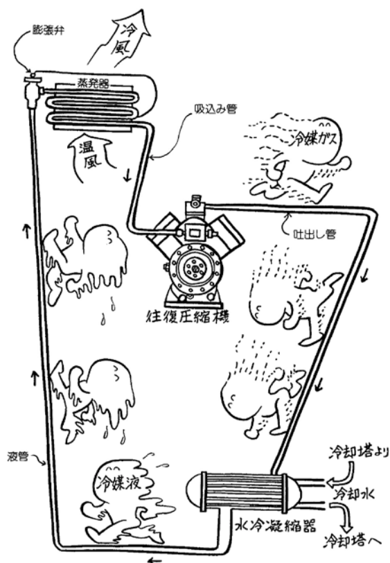
図 圧縮式冷凍機のしくみ（参考文献 [30], p. 101）
