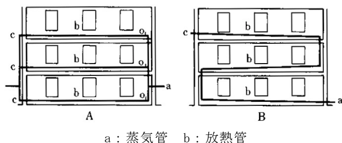
図 同径の鋳鉄管を連続して用いた一管式蒸気暖房 (参考文献 [9], p. 65)
