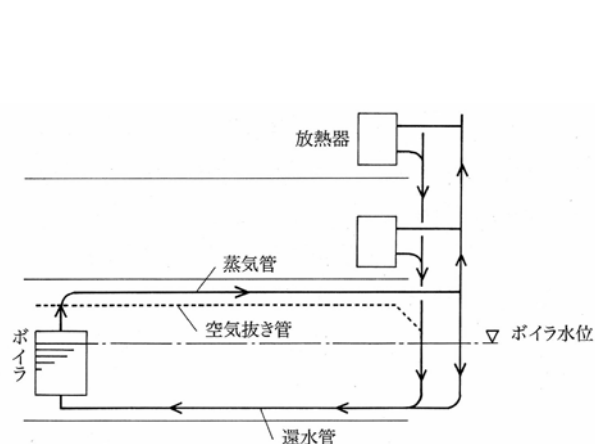
ケルチング式蒸気暖房の模式図 (参考文献 [20], p. 11)
